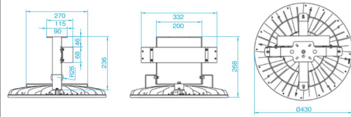
TU-03：吊下げ型アームC (1000用)／寸法図
