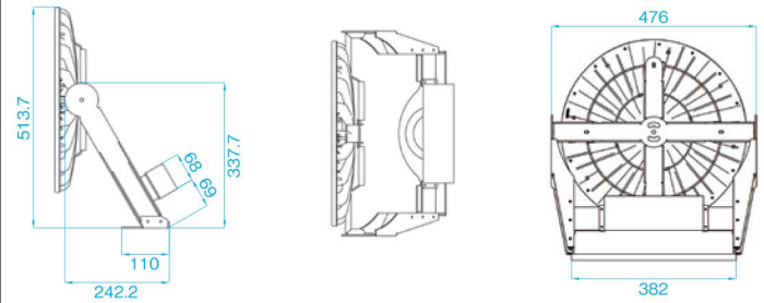
NA-03：投光器型アームC (1000用)／寸法図
