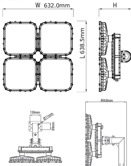
外形寸法図
